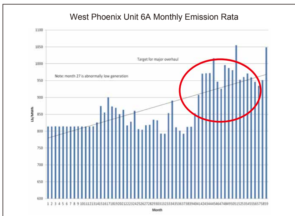
図10 ウェスト・フェニックス6A号機の月単位の排出割合 出典：USEPA大気市場プログラムデータ
