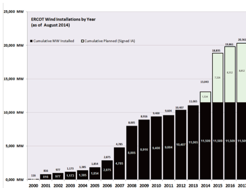
図3 テキサス州の系統運用機関ERCOTの風力発電の導入量 14
