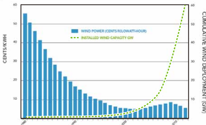
図4 アメリカにおける風力発電のコスト低下 出典：アメリカ風力エネルギー協会 16
