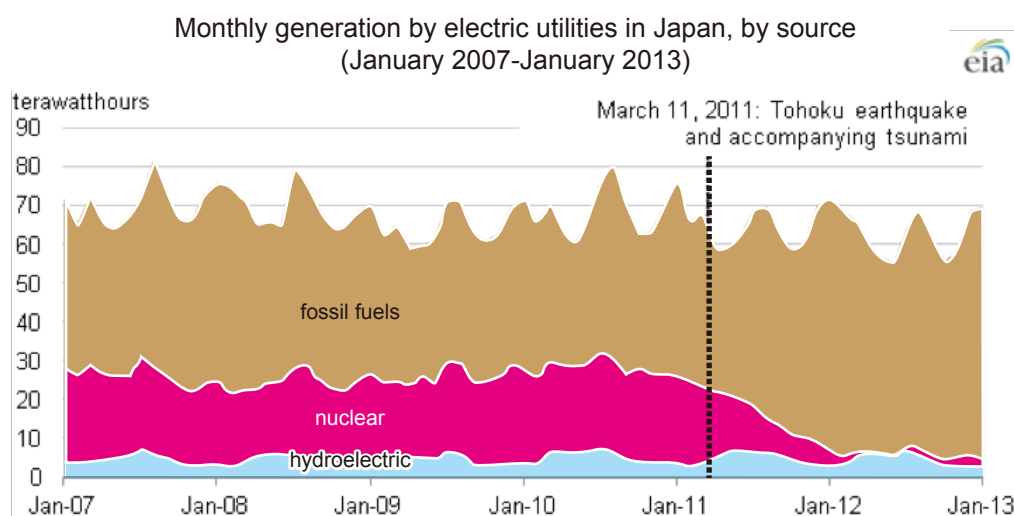
図1 電気事業者による月ごとの発電量（燃料別） 出典：EIA 2
