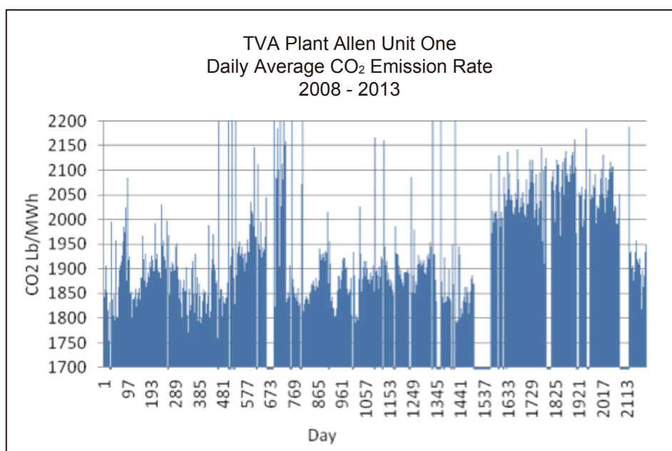
図9 TVA発電プラント・アレン1号機の2008～2013年の日平均CO 2 排出量 出典：EPA大気市場プログラムデータ
