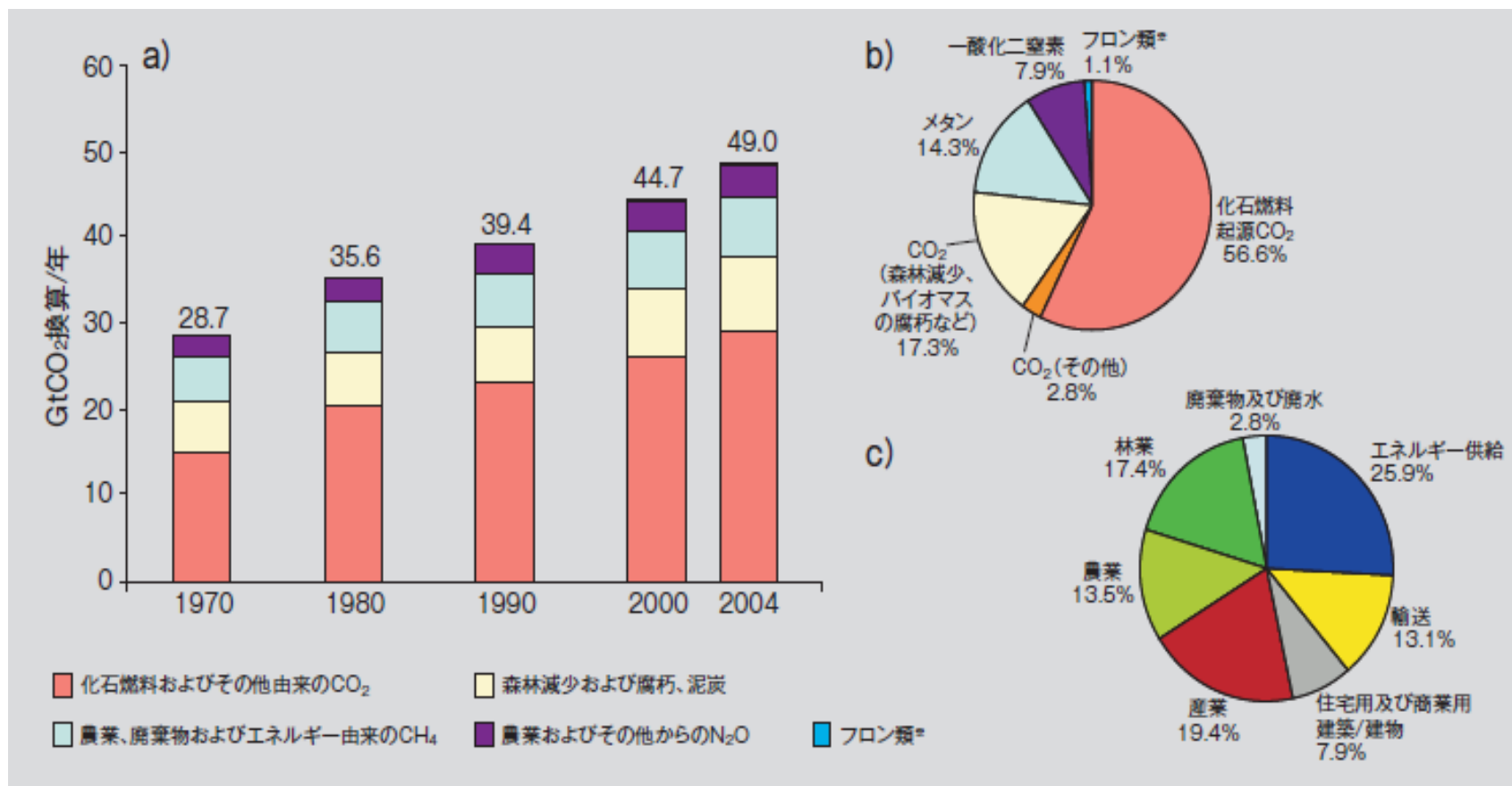
図 SPM.3. (a) 1970~2004年の世界の人為起源温室効果ガスの年間排出量 5 、(b) 2004年の人為起源温室効果ガス総排出量に占めるガス別排出量の内訳 (CO 2 換算ベース)、(c) 2004年の人為起源温室効果ガス総排出量に占める部門別排出量 (CO 2 換算ベース)の内訳。(森林部門には森林減少を含む) [図 2.1]
